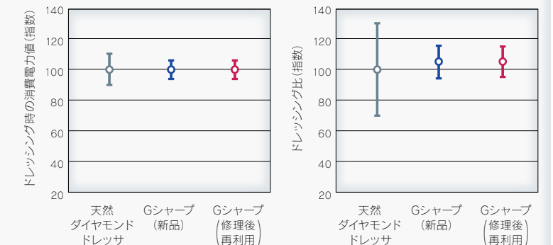
図14 試験結果
