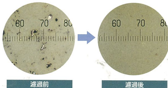
ベアリング超仕上げ加工 (油性) (30 \mu m/10目盛)
